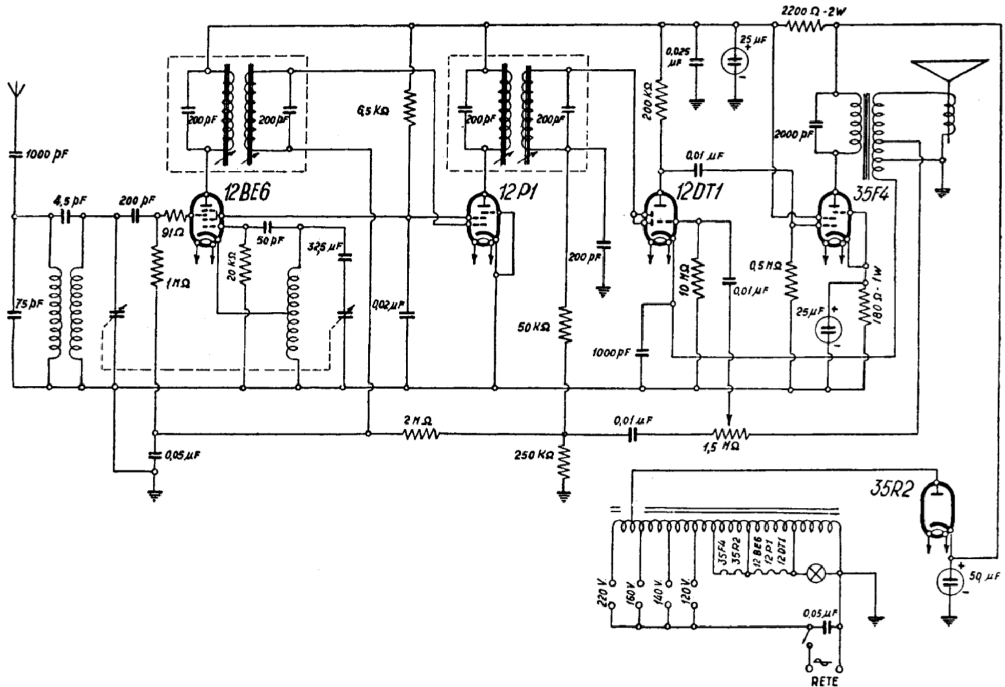
MAGNADYNE RADIO - Mod. A 3 e K 403. Ricevitore a onde medie. Media frequenza a 471 kc/s. Potenza d'uscita 2 watt.
